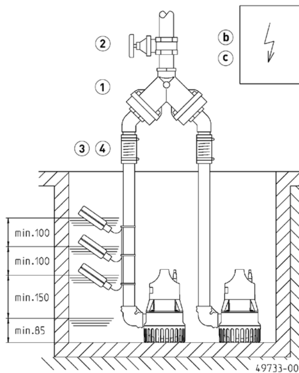
Inbouwvoorbeeld dubbelpomp installatie
