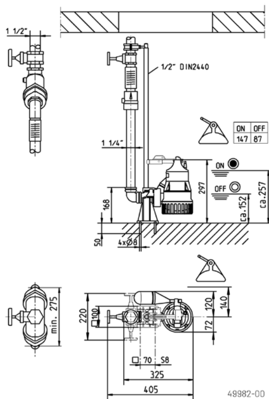
Afmetingen en schakelhoogtes GR 32 (mm)
